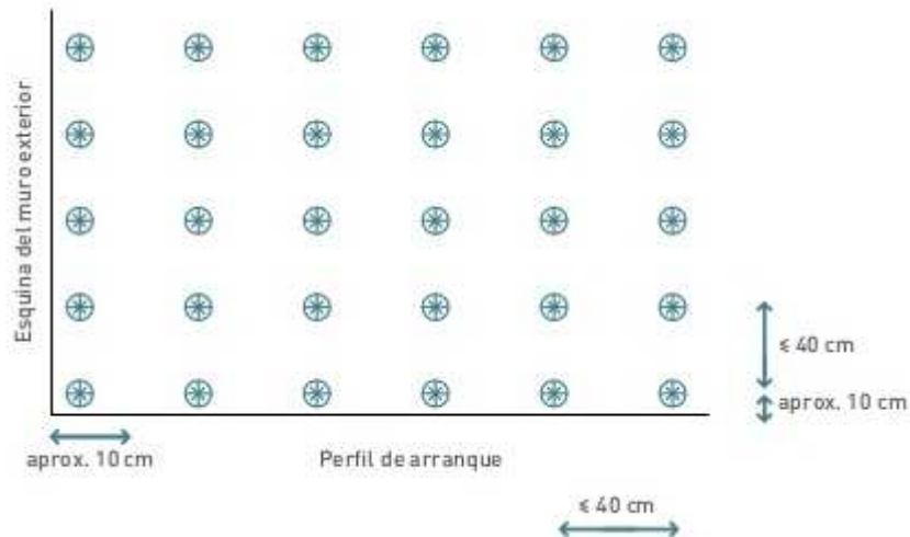
Figura 18. Esquema de la fijación mixta
