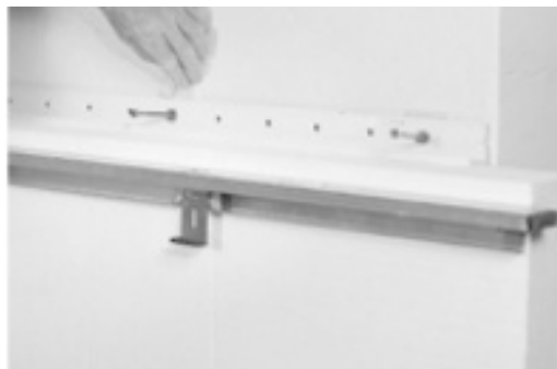
Figura 16. Fotografía de la instalación de un listón de retención.
