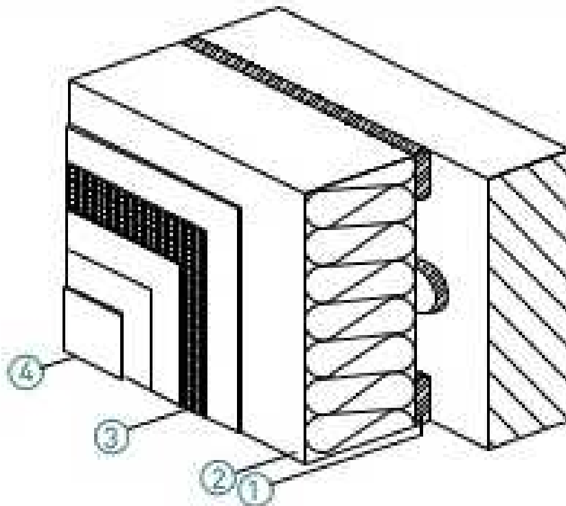
Figura 1. Esquema básico de sistema SATE.
