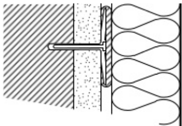
Fotografía 17. Sección constructiva de la fijación mixta
