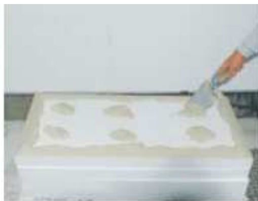
Pegado borde-punto en una plancha de EPS
